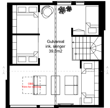
PLAN LOFT
