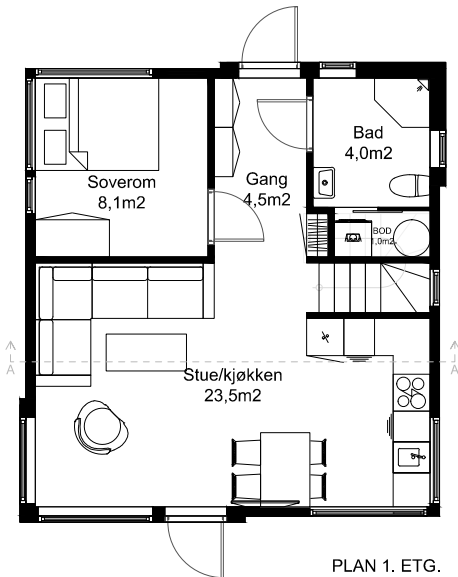
PLAN 1. ETG.
