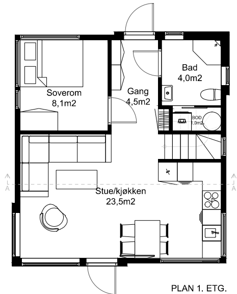
PLAN 1. ETG.
